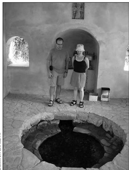
Jedno z wywierzysk w klasztorze Sv. Naum, Macedonia.
