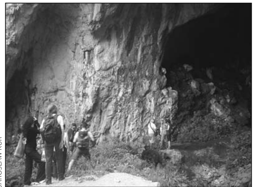
Stanowisko archeologiczne w Turzii Gorges
